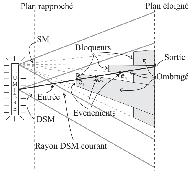
FIG. 3.1 – Un rayon correspond à un seul pixel du PDSM . Le rayon du PDSM est utilisé pour accumuler l'information d'atténuation calculée à partir du shadow map d'un échantillon. Les événements d'ombre ( e_1, e_2, e_3 , arrière-plan) sont insérés dans ce pixel du PDSM .
