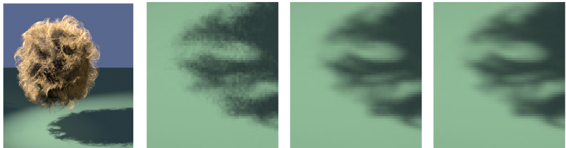
FIG. 2.13 – Deep shadow map . De gauche à droite : Boule de 50 000 cheveux, shadow map de 512 \times 512 , shadow map de 4096 \times 4096 , DSM de 512 \times 512 (image tirée de [LV00]).
