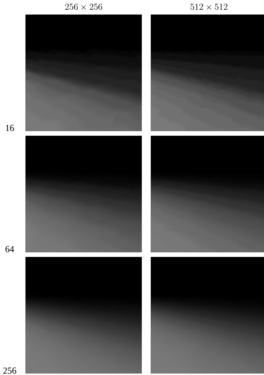
FIG. 4.6 – Résultats pour différentes résolution de PDSM (non compressés) et différents nombres d'échantillons. Colonne de gauche : PDSM de 256 \times 256 , à droite : 512 \times 512 . De haut en bas : 16 échantillons, 64 échantillons et 256 échantillons (se référer à la figure 4.5 pour l'image complète).
