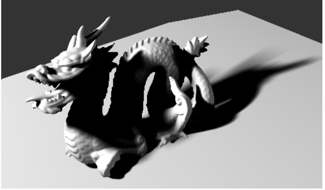
FIG. 3.6 – Rendu du modèle de Dragon de Stanford avec un PDSM de 512 \times 512 et 256 échantillons.
