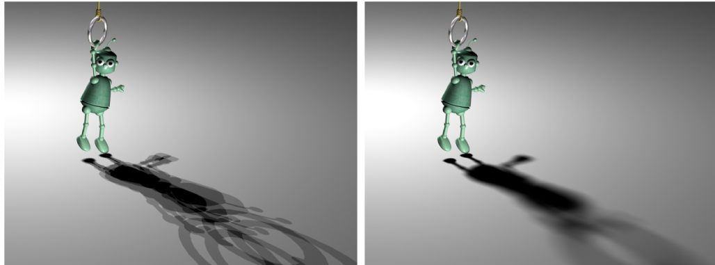
FIG. 2.11 – Effet d’un nombre différent d’échantillons sur la lumière. Gauche : 4 échantillons. Droite : 1024 échantillons (image tirée de [HLHS03]).
