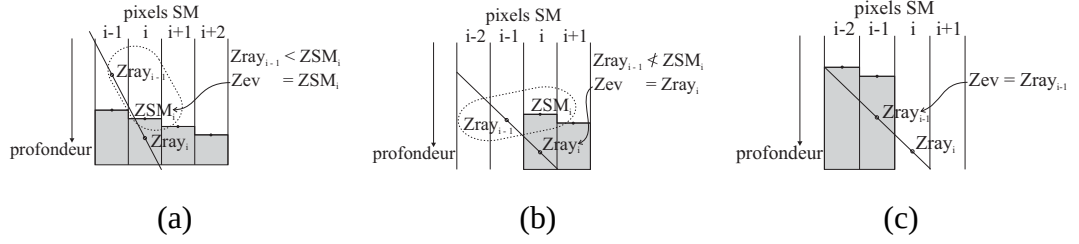
FIG. 3.4 – Les pixels du shadow map correspondent aux régions verticales i-2 , i-1 , i , etc. ; les points représentent l'information de profondeur au centre de chaque pixel du shadow map ; la profondeur du rayon du PDSM croît en traversant le shadow map . Choix entre la profondeur du rayon du PDSM et celle du shadow map au pixel i : (a) la profondeur du shadow map est correcte, (b) la profondeur du shadow map est incorrecte, (c) illustration du choix de la profondeur du pixel précédent pour les événements de sortie.
