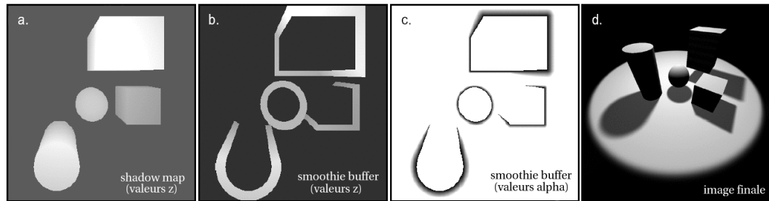
FIG. 2.9 – Algorithme des smoothies . (a) Création d'un shadow map standard. Puis, construction de primitives ( smoothies ) aux silhouettes. (b) Rendu des smoothies dans un tampon de profondeur. (c) Pour chaque pixel du smoothie buffer , stockage d'un alpha qui dépend du ratio de distances entre la source de lumière, le bloqueur et le receveur. (d) Finalement, rendu de la scène du point de vue de la caméra avec comparaison avec les valeurs du shadow map et du smoothie buffer (image adaptée de [CD03]).
