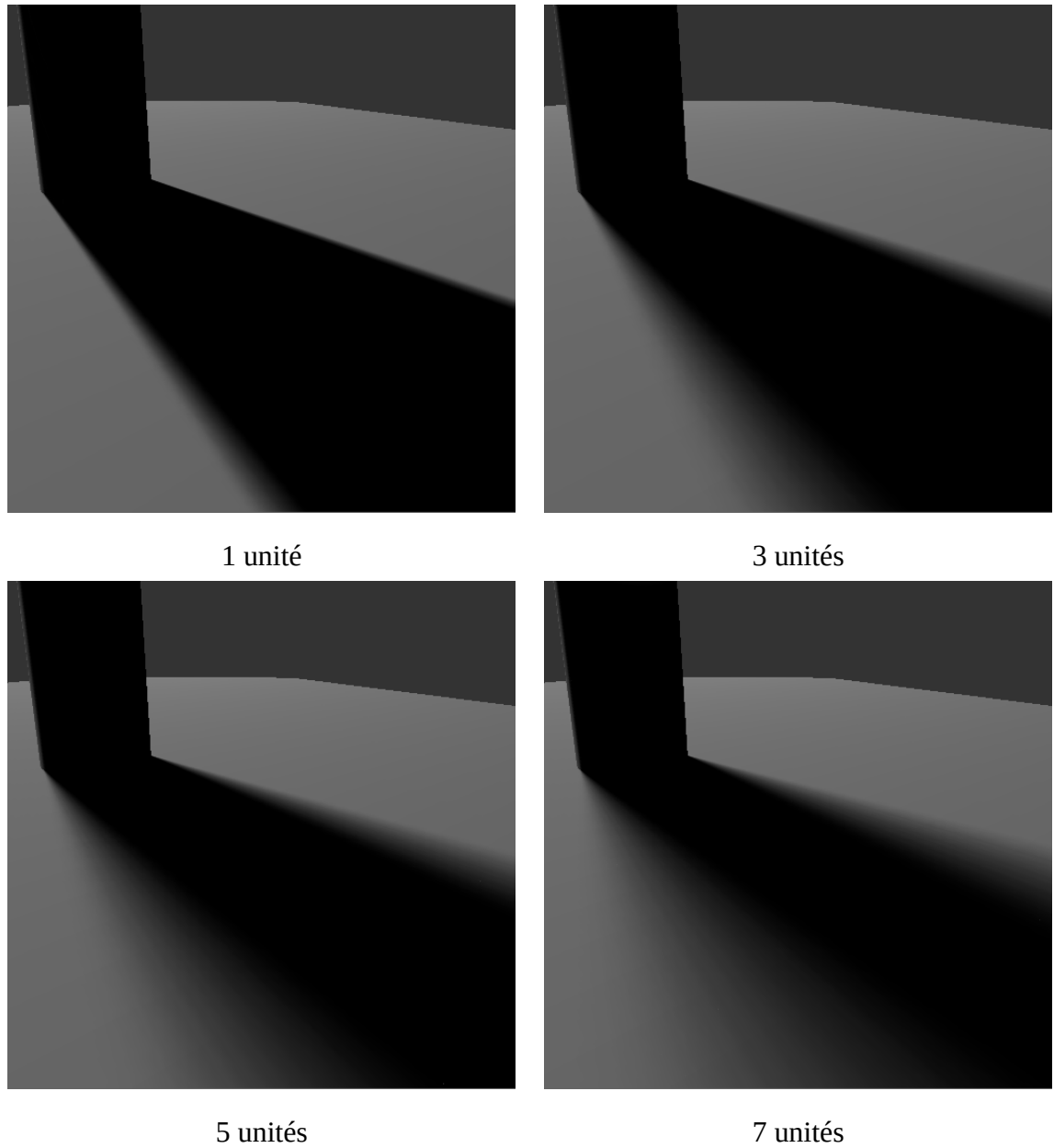
FIG. 4.7 – Résultats pour différentes tailles de source de lumière ( PDSM de 512 \times 512 , 256 échantillons). Le cylindre a un rayon de 1 unité.
