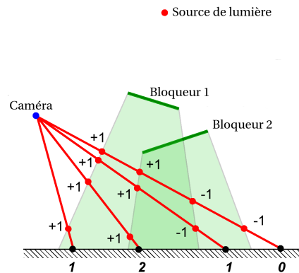
FIG. 2.2 – Illustration en 2D des volumes d’ombre (image adaptée de [HLHS03]).
