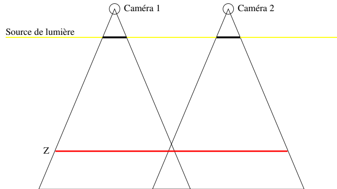
FIG. 3.5 – Tous les points le long de la ligne Z ont la même profondeur, tant dans la caméra de la vue 1 que de la vue 2.
