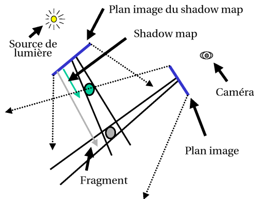
FIG. 2.7 – Diagramme illustrant l'algorithme de shadow mapping .
