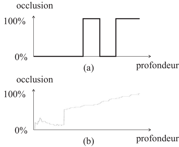
FIG. 3.2 – (a) Visibilité le long d'un rayon pour un échantillon. (b) La fonction d'atténuation finale le long du rayon du PDSM , i.e. , la somme des contributions de chacun des shadow map échantillons. Il est à noter que cette fonction n'est pas strictement croissante, contrairement à Lokovic et Veach [LV00].
