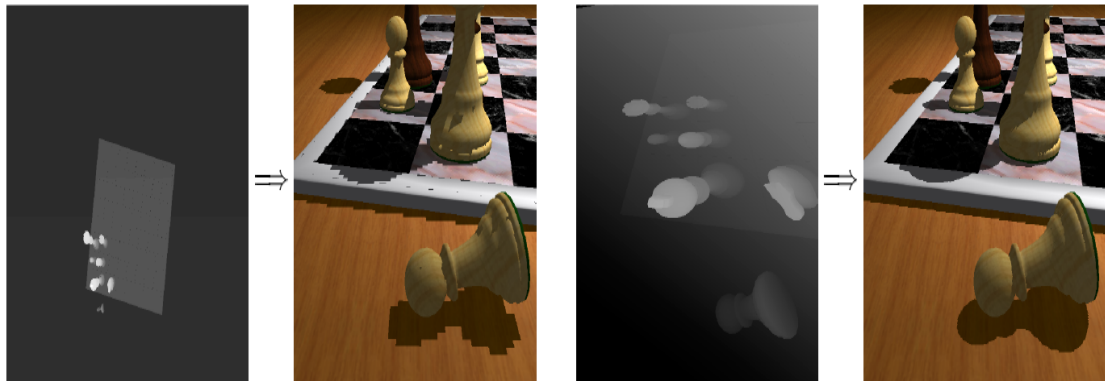
FIG. 2.8 – Le tampon de profondeur en espace perspective. À gauche, un tampon de profondeur traditionnel avec ses problèmes d’aliasage. À droite, en espace perspective (image tirée de [SD02]).
