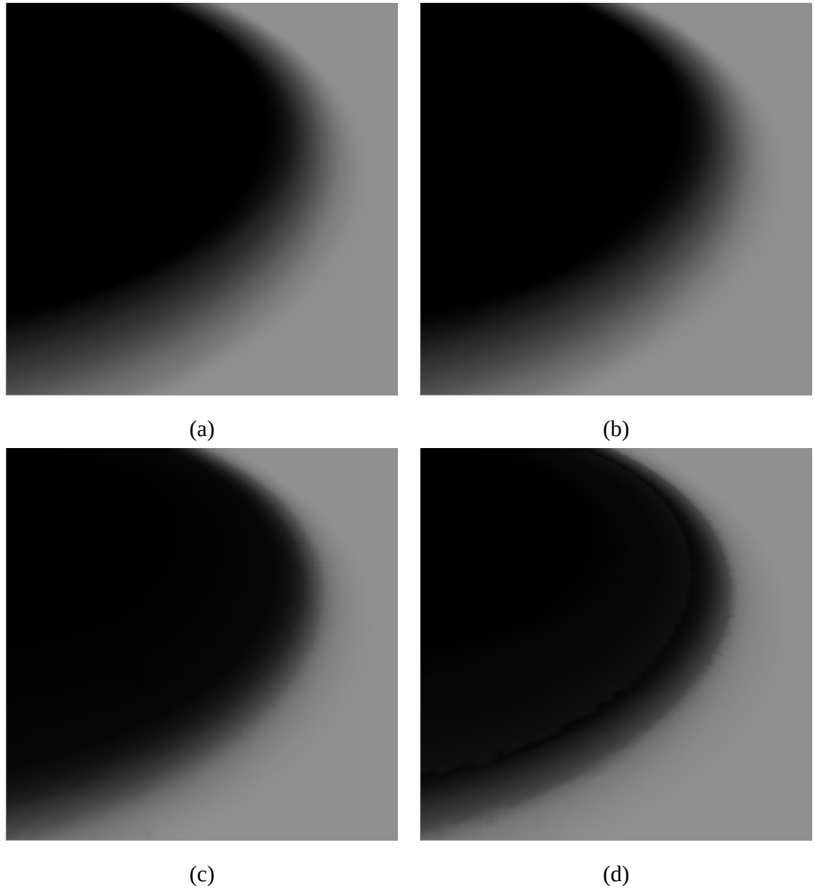
FIG. 3.8 – Impact visuel des différents niveaux de compression : (a) Aucune compression, (b) 2% d’erreur autorisé, (c) 5% et (d) 10%. La différence est particulièrement notable aux frontières de la pénombre dans les deux dernières images.
