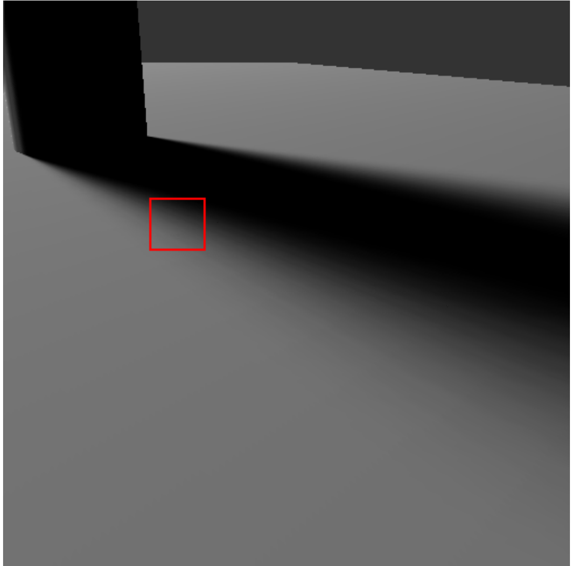
FIG. 4.5 – Rendu d'un cylindre ( PDSM de 512 \times 512 avec 256 échantillons). Le rectangle rouge est grossi dans la figure 4.6.
