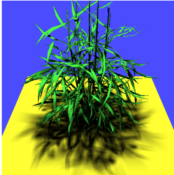
FIG. 2.12 – Layered attenuation map (image tirée de [ARHM00]).
